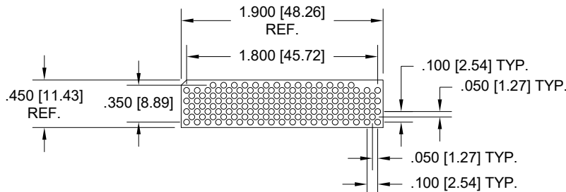
Fig. 24 144 Pins Thru-Hole: 585-19-25-144-211S-R27-BT14 Surface Mount: 585-19-25-144-384S-R27-BT14
