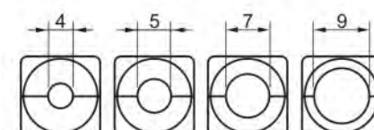
Grommet Sizes - MHDSCK:
