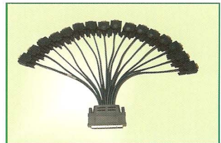
HD200P(4ROWS)+DB9M x16
