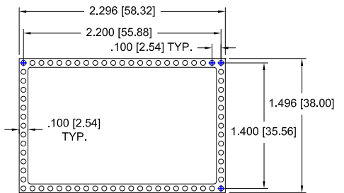
Fig. 62 72 Pins
